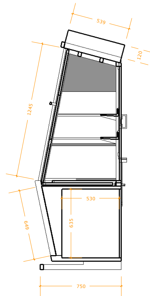
A :: SECTION A03 scale: 1:20
