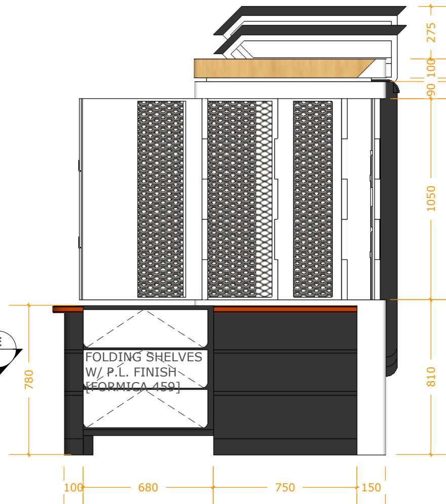
D :: BACK ELEVATION scale: 1:20
